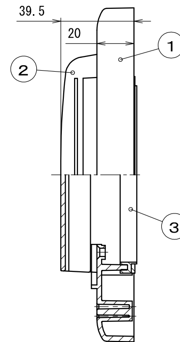
A-A断面図
